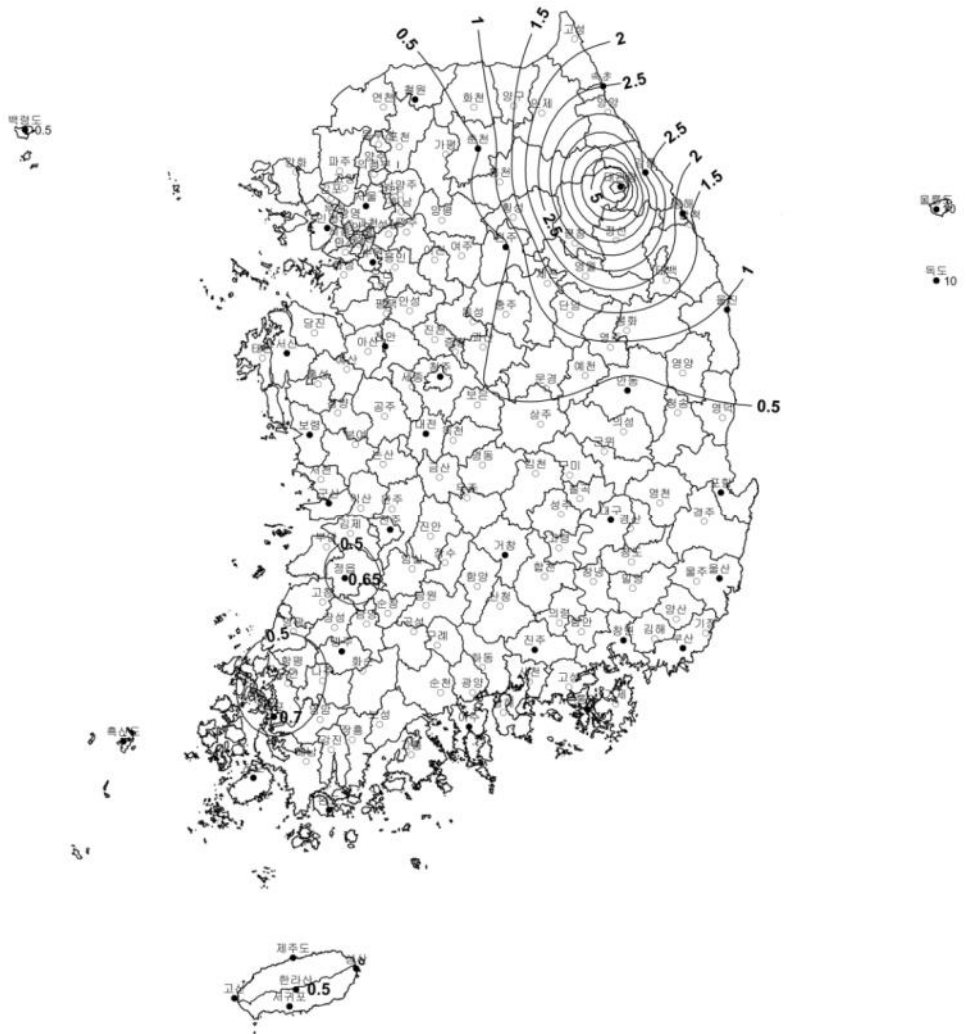
<그림 0304.2.1> 기본지상적설하중 S_g
