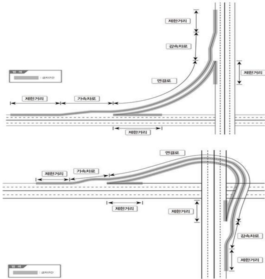
<예시도> 입체교차로의 연결 금지구간
